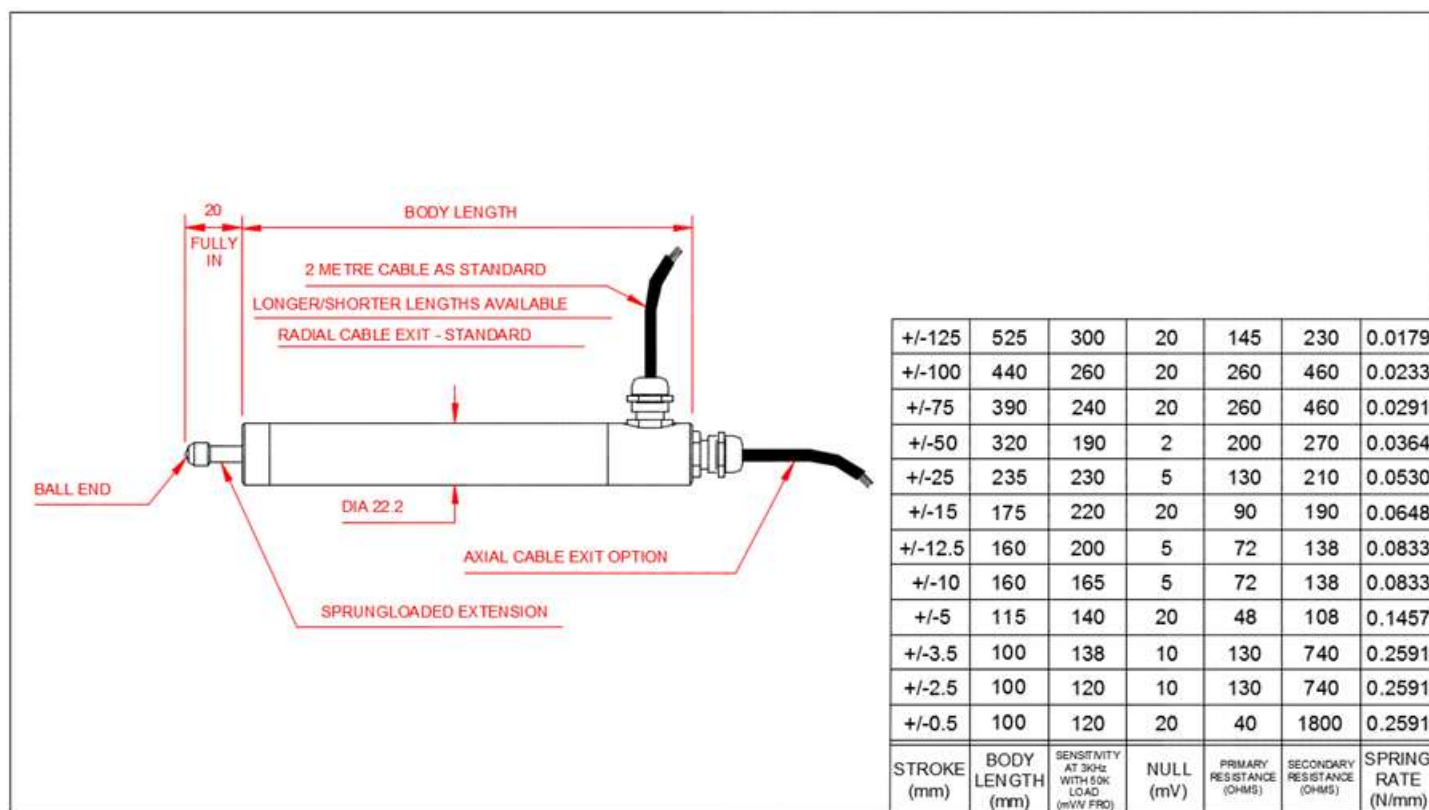
外形寸法図
