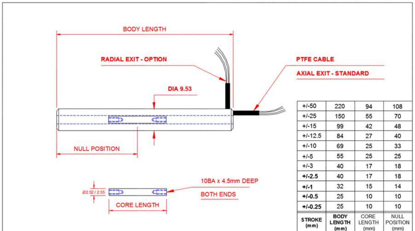
外形寸法図
