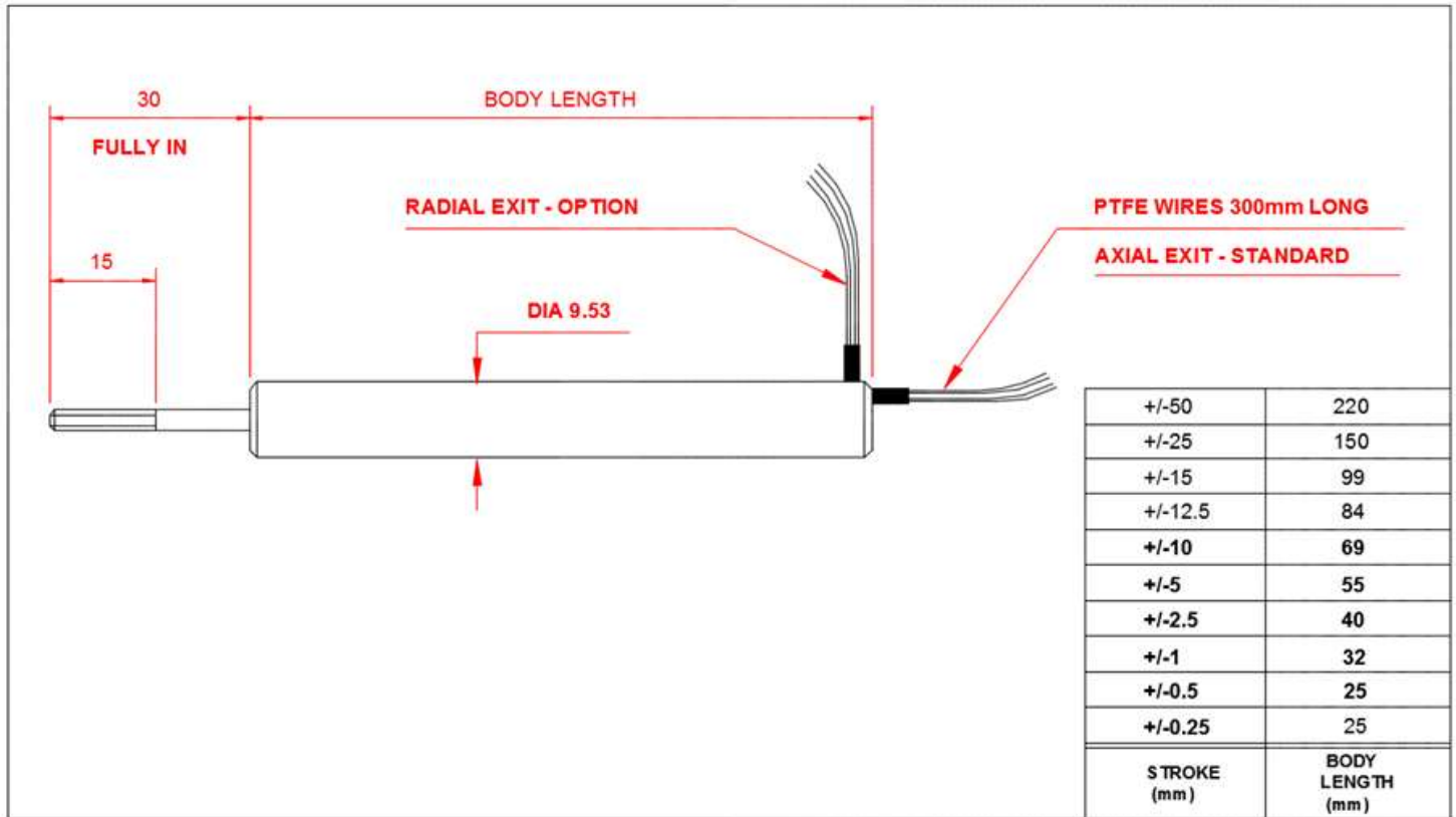
外形寸法図
